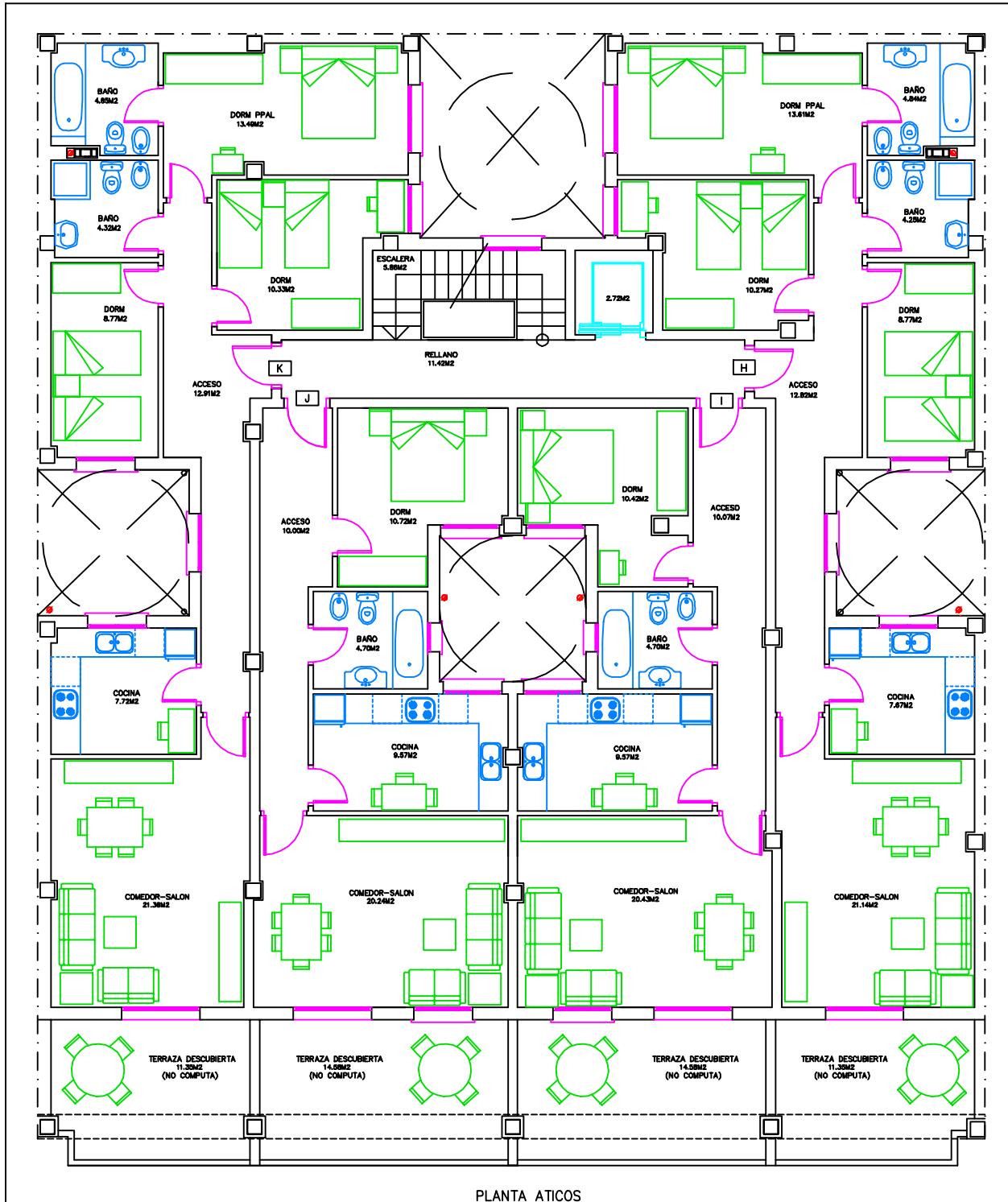
PLANTA ATICOS
